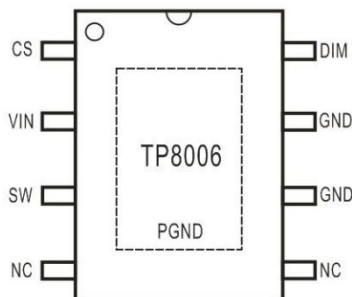
ESOP8L
