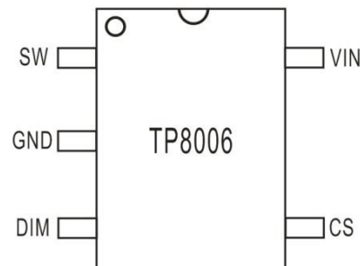
SOT23-5L
