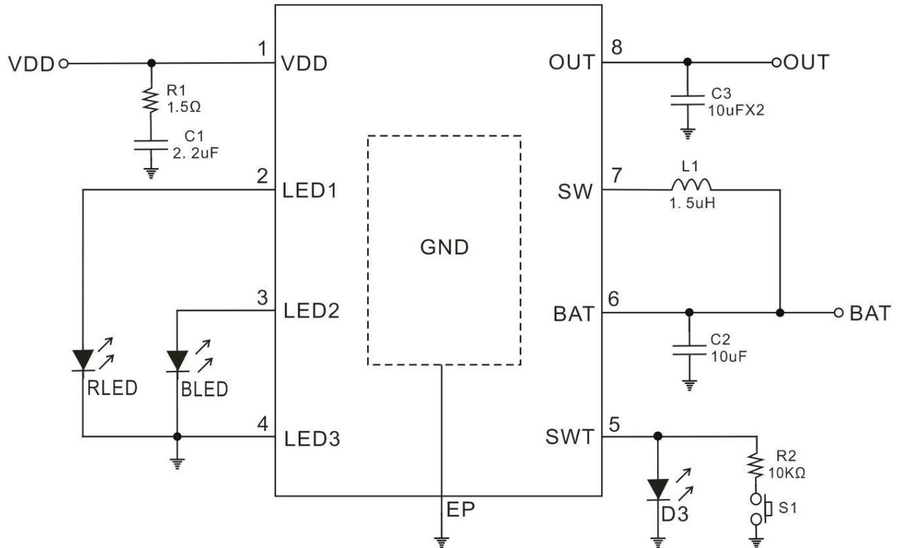
2LED 指示灯典型应用电路
