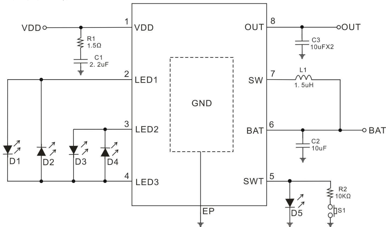
4LED 指示灯典型应用电路
