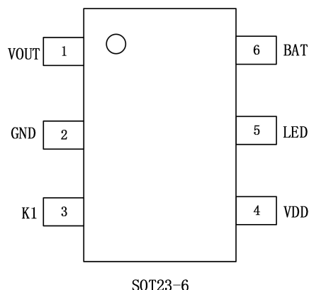
SOT23-6
